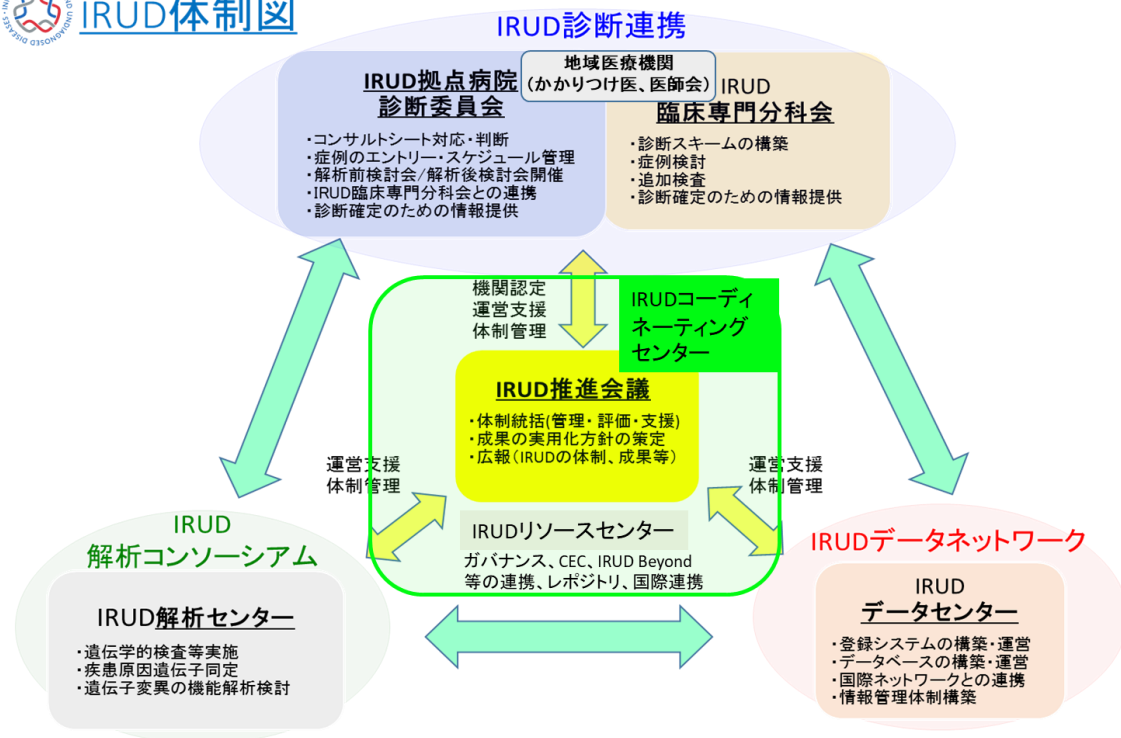
図1 IRUD体制
